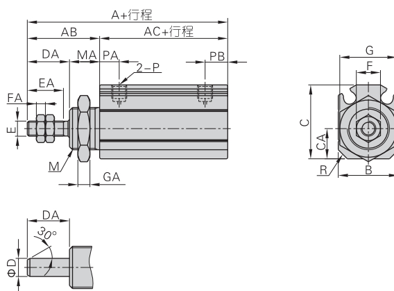
無牙型活塞杆
