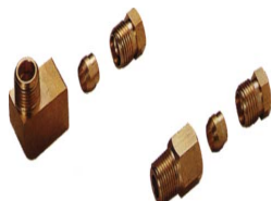
潤滑油管路專用直、L型接頭
