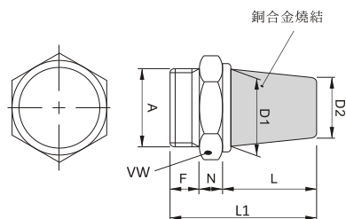
SCSL-L長頭型銅消音器
