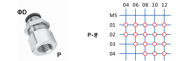
SPMF 隔板內牙直接頭
