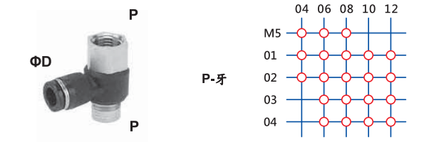
SPHF L 型 - 短內外牙三通
