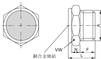
SCSL平頭型銅消音器
