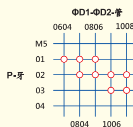
SPTKD 異徑外牙五通
