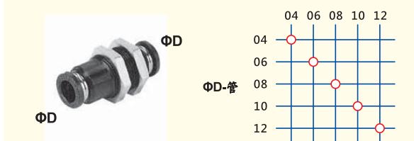
SPMM 隔板直通
