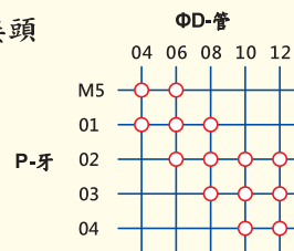
SPHY L 型 - 短外牙 Y 型三通
