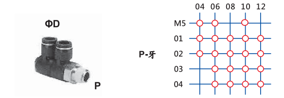
SPHH L 型外牙三通
