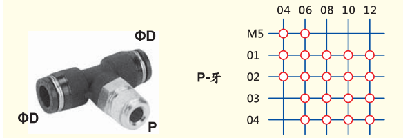
STT T 型外牙三通
