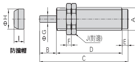
外型尺寸圖
